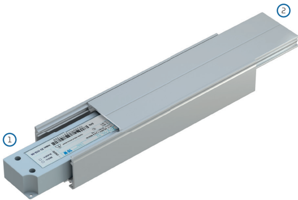
Schemat złożenia elementów systemu oświetleniowego przy wykorzystaniu profilu INSO wpuszczanego oraz (1) zasilacza LED, (2) profilu montażowego MODI Assembly scheme for elements of the lighting system using INSO recessed profile and (1) LED power supply, (2) MODI mounting profile
